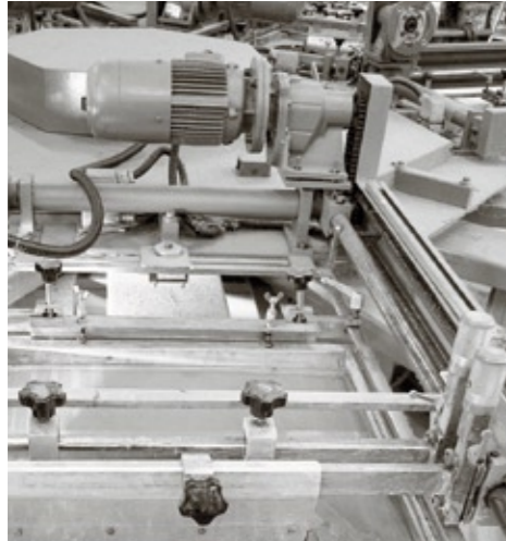
▲ Sérigraphie flock
